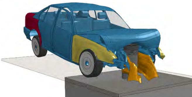
Simulation eines Anpralls durch ein Rammfahrzeug.
